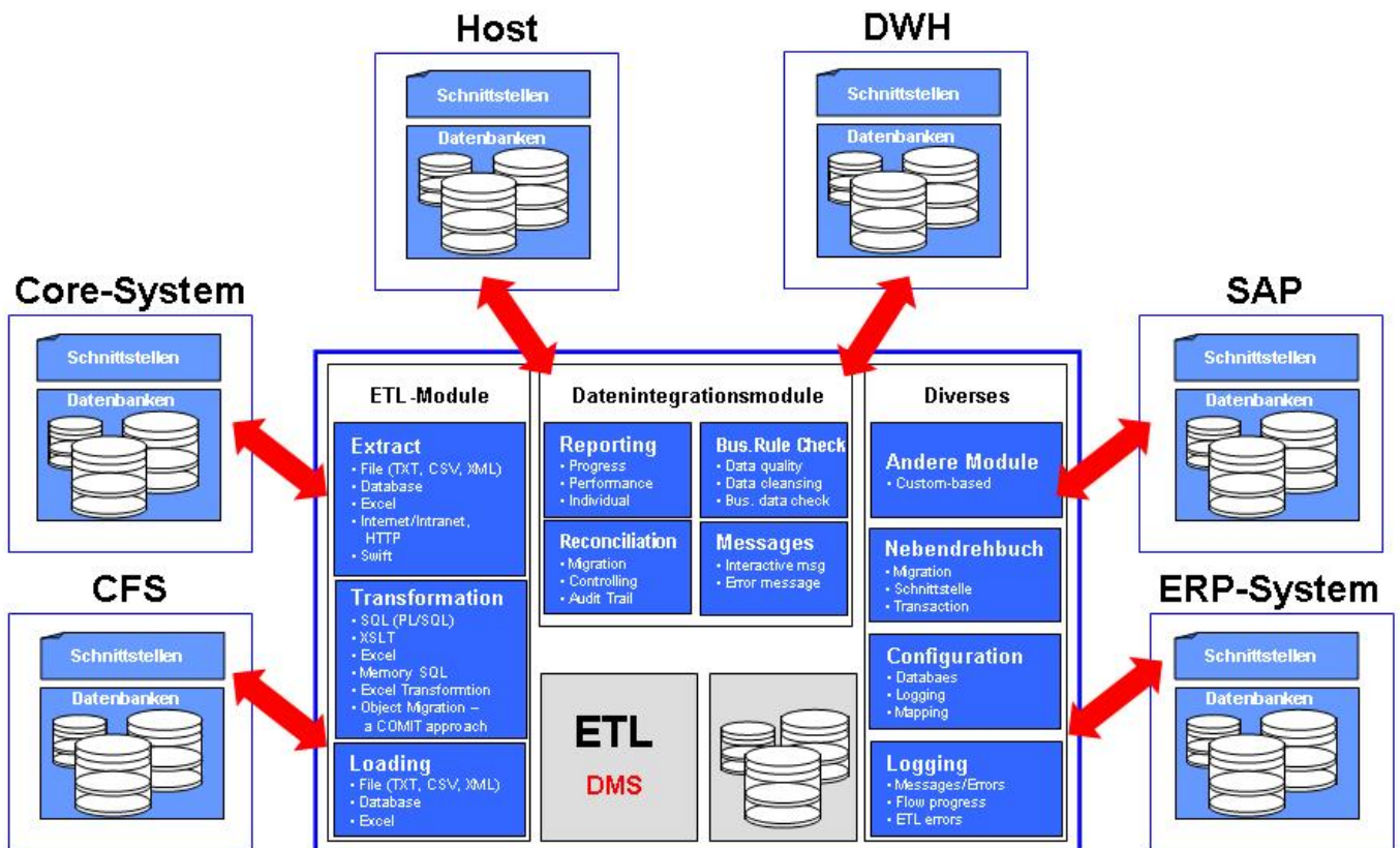
Datenintegrations-Framework (modularer Aufbau)
